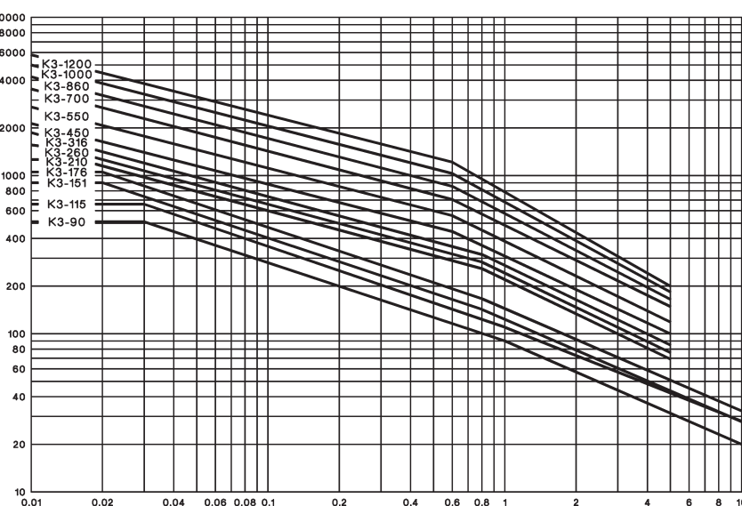
Millionen Schaltspiele
