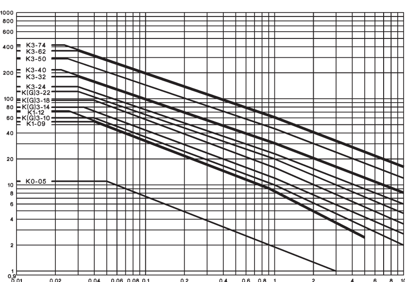
Millionen Schaltspiele
