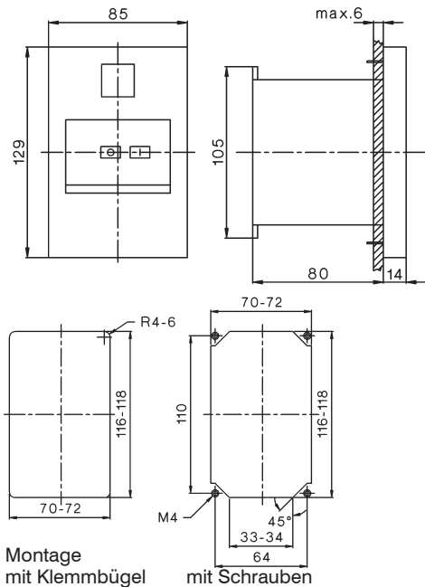
Isolierstoff-Frontplatte MU25A-C55
