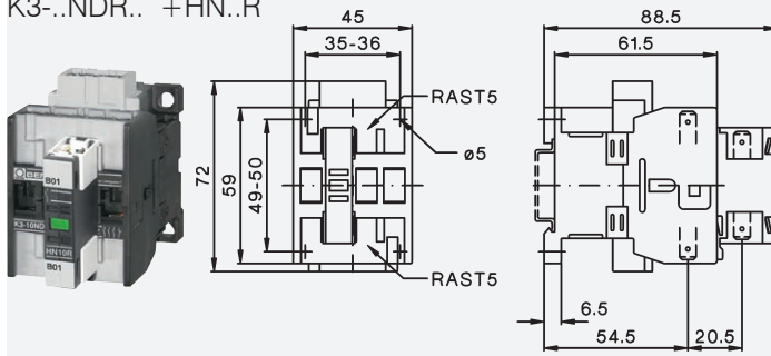
K3..NDR.....PZ + U3/32..
