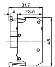
All dim. ± 0,2
