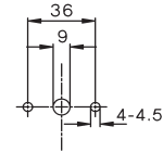
Bohrplan
