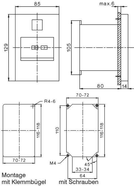
Isolierstoff-Frontplatte MU25A-C55
