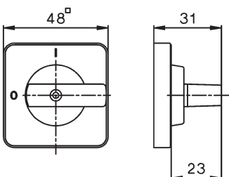
Schild 48 Griff
