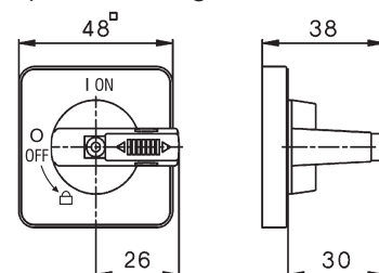
Sperrvorrichtung SV1.
