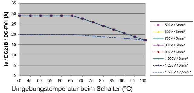
Schalter offen LS16..., 4 Kontakte in Serie + 2 parallel (A4+2)
