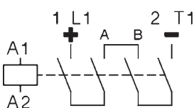
Schaltbild (4 Kontakte)
