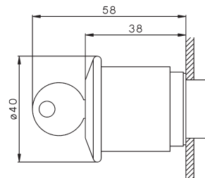
Pilz-Druck-Zug-Taster Ø40mm mit Schlüssel
