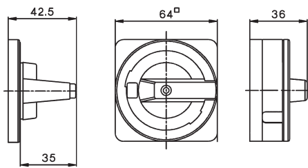
Sperrvorrichtung SV4
