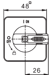
Sperrvorrichtung SV1
