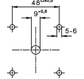
Bohrplan Montageschraube S3631N M=1,2-1,4 Nm
