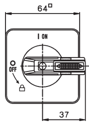
Sperrvorrichtung SV1
