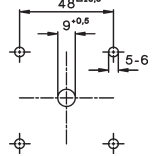
Bohrplan Montageschraube S3631N M=1,2-1,4 Nm
