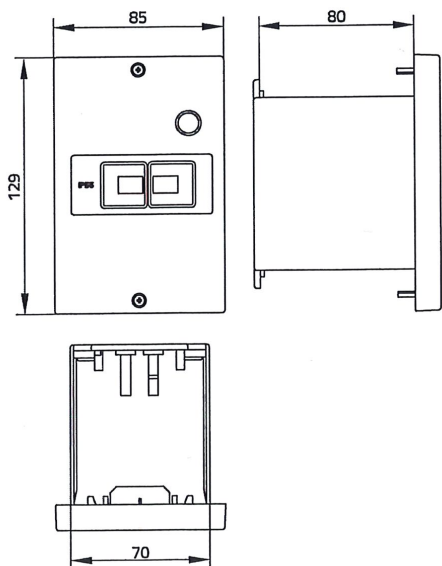
Isolierstoff-Frontplatte MU25-C55
