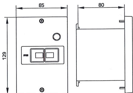
Isolierstoff-Frontplatte MU25-C55
