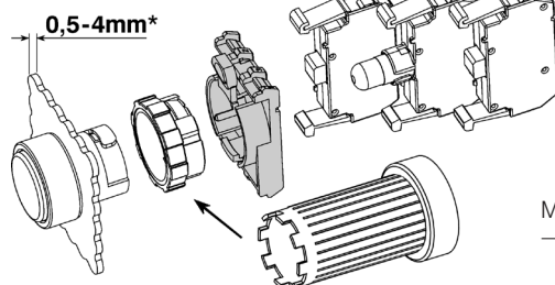
Kuppelstück B3M
