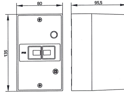
Isolierstoffgehäuse MU25-O55
