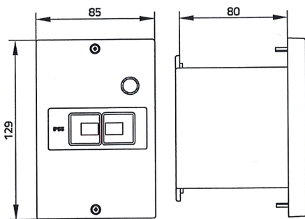
Isolierstoff-Frontplatte MU25-C55
