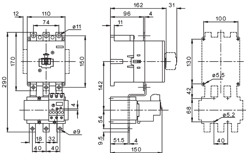
Bohrplan
