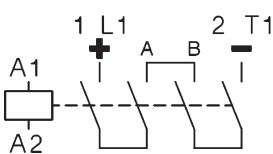
Schaltschema (4 Kontakte)
