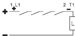
Anschluschema 1-polig
